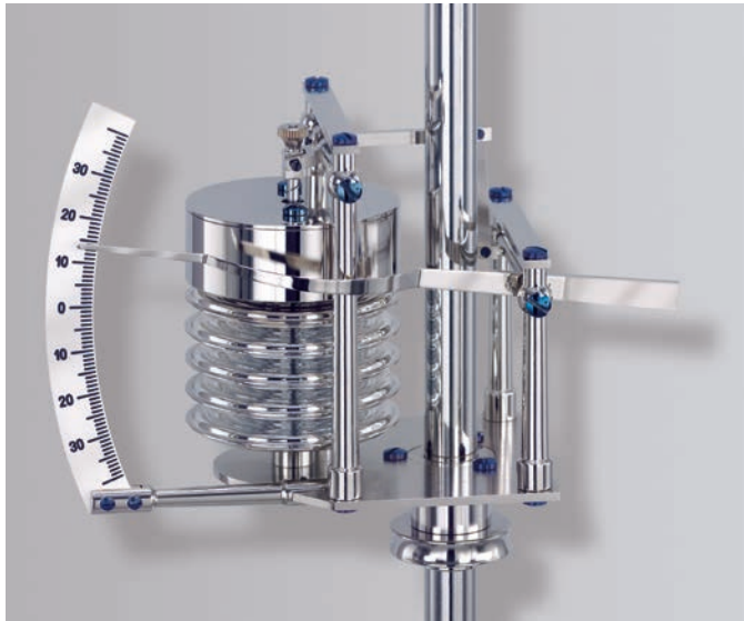
Um größeren Gangabweichungen durch Luftdruckschwankungen vorzubeugen, ist am Pendel ein Aneroidoseninstrument mit Barometeranzeige angebracht. To prevent major accuracy deviations as a result of fluctuations in air pressure, an aneroid barometric compensation is added to the pendulum.
